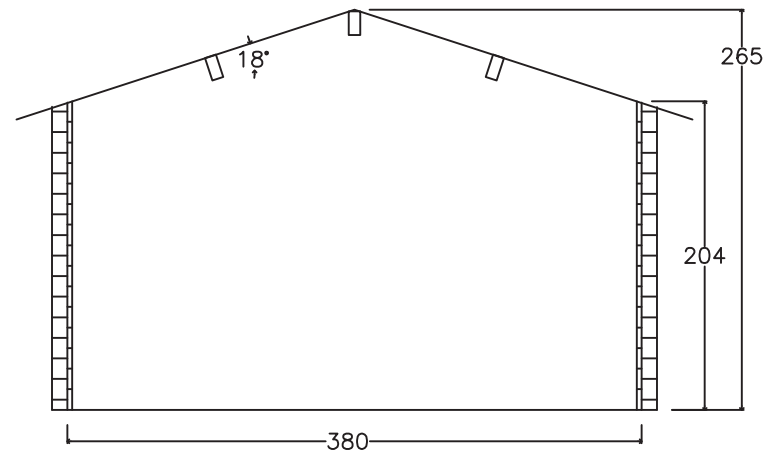
Schnitt / profile
