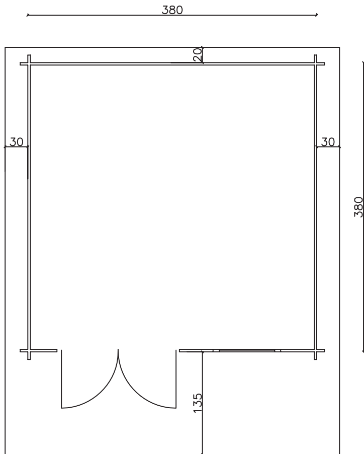
Grundriss / ground plan plattgrund / plan / rzut
