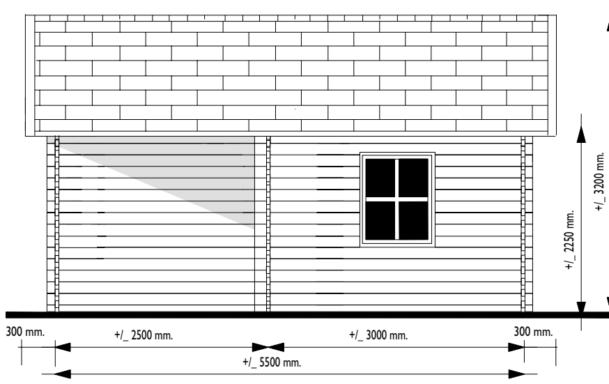
Zij aanzicht Seiten Ansicht Side view
